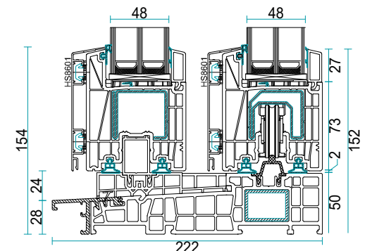
Salamander EvolutionDrive 82 Aluscale
