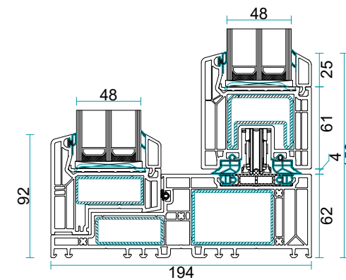
Vekamotion 82 MAX
