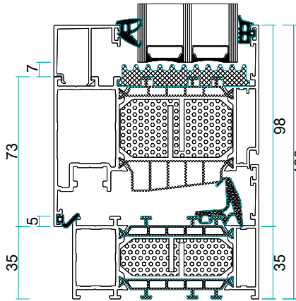
Aliplast Genesis 90
