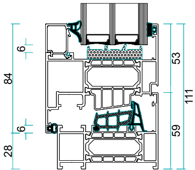
Aluprof MB-86N
