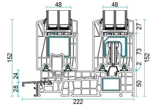
Salamander EvolutionDrive 82
